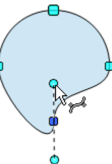
Abbildung 19: Eine Tangente drehen
