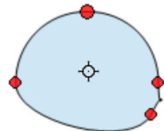
Abbildung 30: Ergebnis der Drehung
