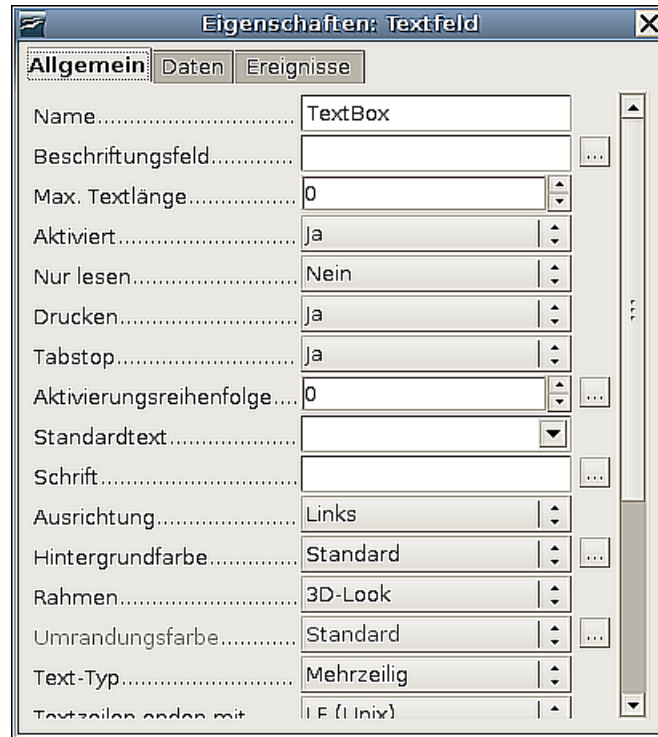
Abbildung 2: Die Steuerelement-Eigenschaften
