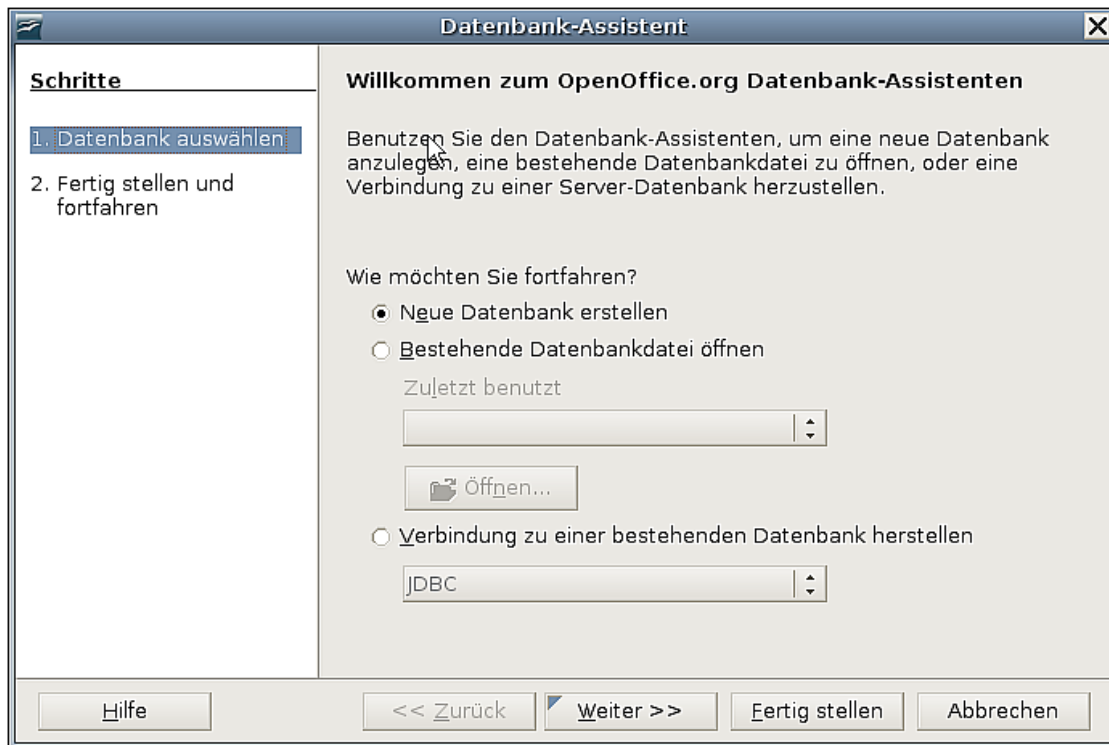
Abbildung 6: Der Datenbank-Assistent
