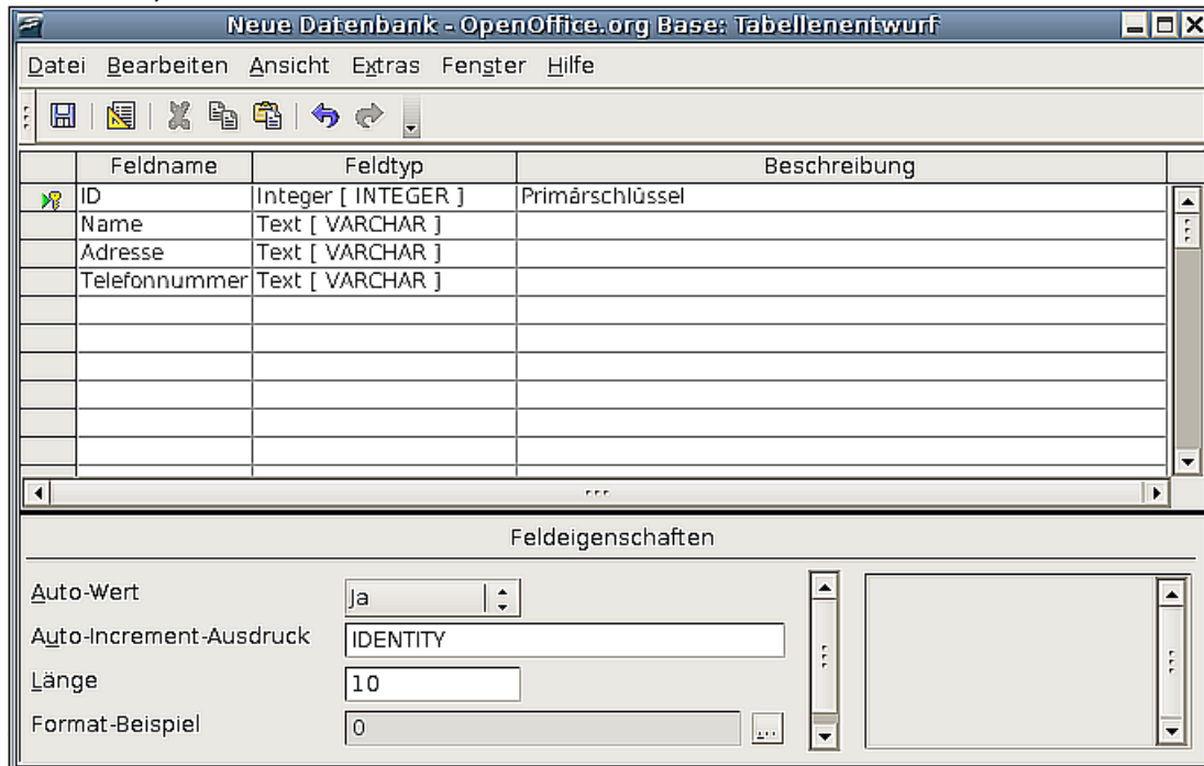
Abbildung 8: Das Tabellenentwurf
